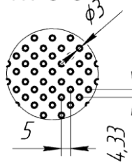
Перфорация Rv 3-5
